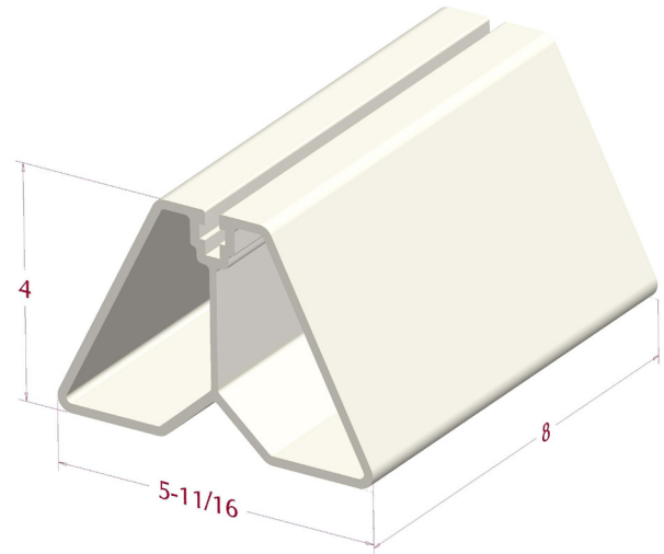
PedestalPlus
